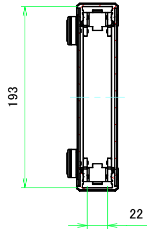
A-A (1:4)
